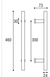
Maniglione singolo Door pull handle
