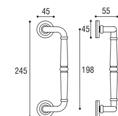
Maniglione zancato Door pull handle
