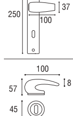
Maniglia con placca rettangolare 8 x 85 yale Door handle with rectangular plate 8 x 85 yale
