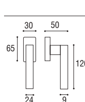
Maniglia per finestra DK 7 x 40 rosetta rettangolare Window handle DK 7 x 40 rectangular rose
