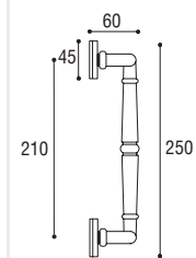
Maniglione singolo Door pull handle
