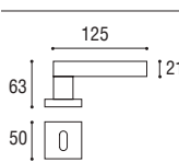
Maniglia con rosetta e bocchetta quadrata Door handle with square rosette and key hole
