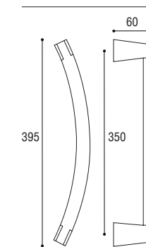
Maniglione singolo Door pull handle
