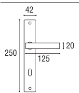
Maniglia con placca rettangolare 8 x 90 Door handle with rectangular plate 8 x 90
