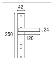
Maniglia con placca rettangolare 8 x 90 Door handle with rectangular plate 8 x 90
