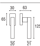
Maniglia per finestra DK 7 x 40 rosetta rettangolare Window handle DK 7 x 40 rectangular rose
