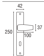
Maniglia con placca rettangolare 8 x 90 Door handle with rectangular plate 8 x 90
