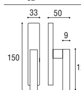
Cremonese EZ con placca rettangolare e impugnatura maniglia Window handle EZ with rectangular plate
