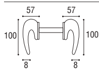
Bilancino 8 per attacco vetro A pair of levers 8 for glass
