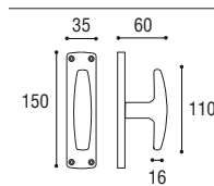
Cremonese EZ Window handle EZ
