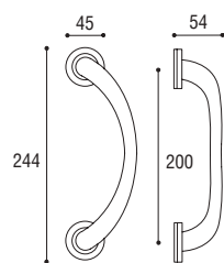
Maniglione singolo Door pull handle
