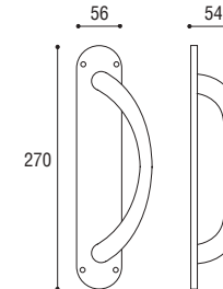
Maniglione singolo su placca ovale con 4 fori Single pull handle on oval plate
