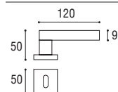
Maniglia con rosetta e bocchetta quadrata Door handle with square rosette and key hole
